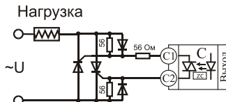
Подключение внешних тириستоров к выходу "С"
